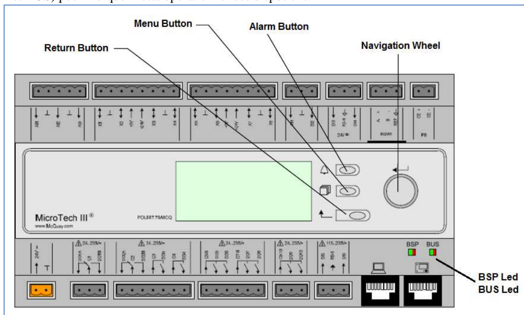
Figure du régulateur "MicroTech III" avec indications des boutons et LED principaux
