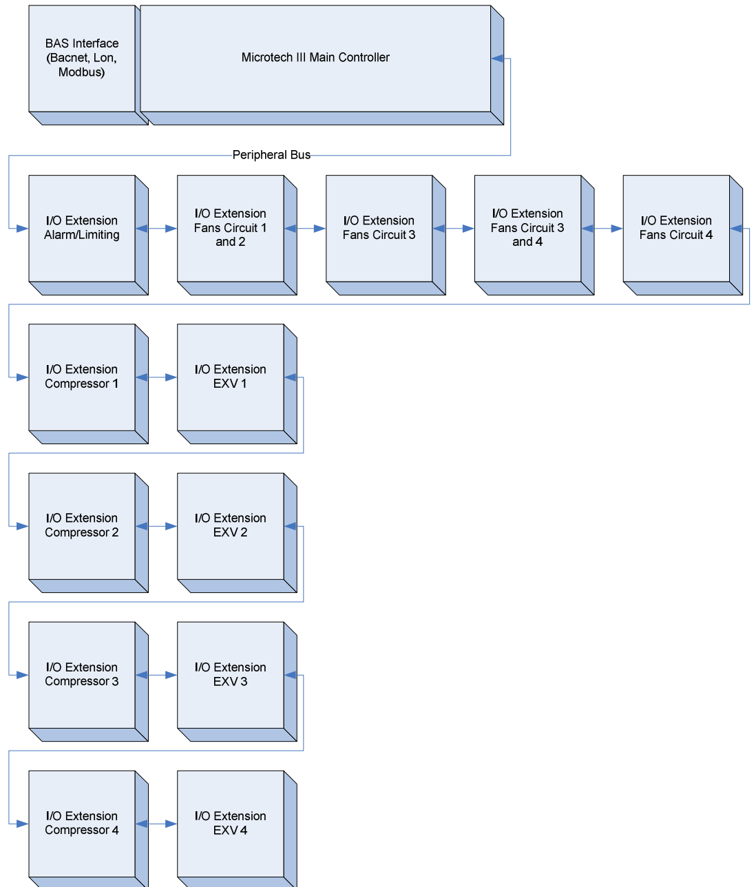
Figura 4, Arquitectura do sistema
